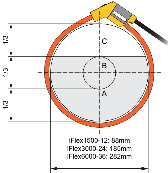
Figure 12. Fenêtre de sonde iFlex
