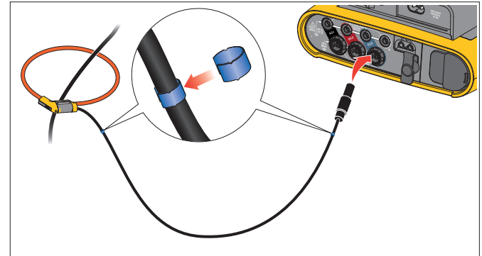
Figure 4. Cordons de mesure avec marqueurs de câbles
