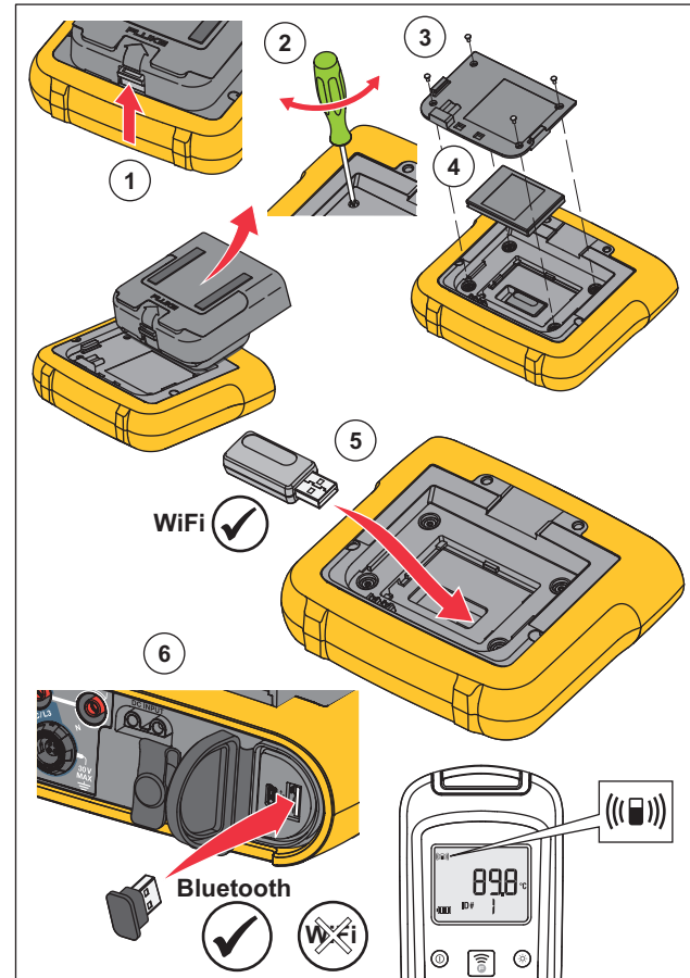
Figure 1. Installation de l'adaptateur
