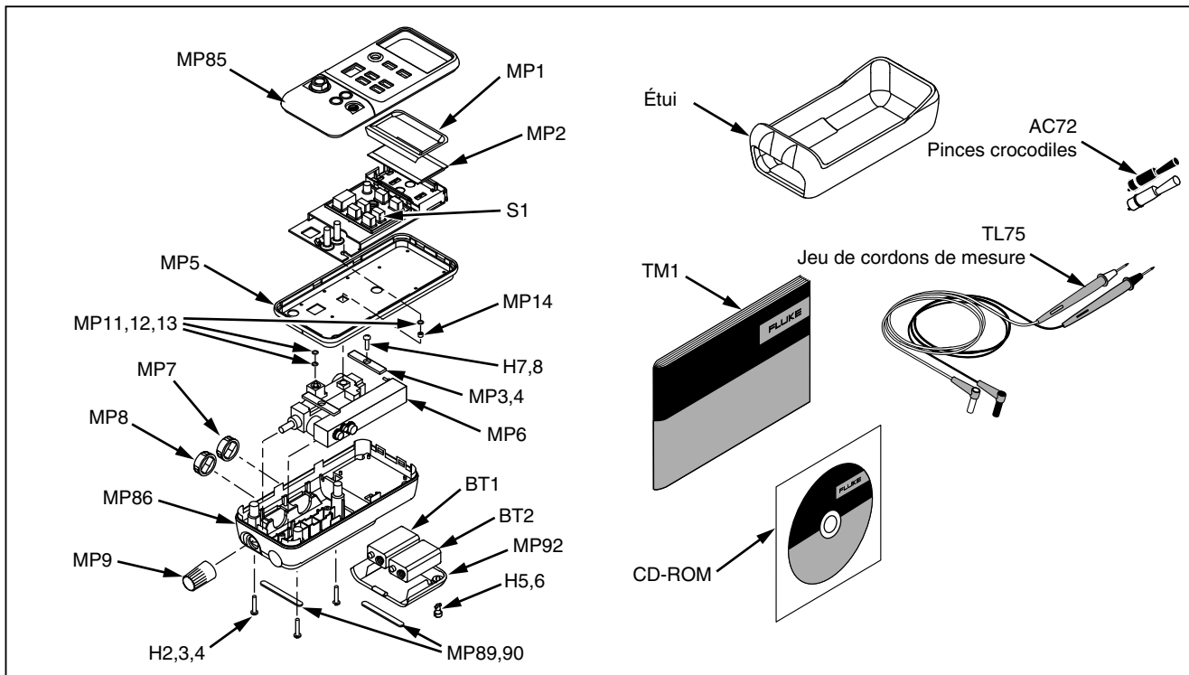
Figure 11. Pièces détachées
