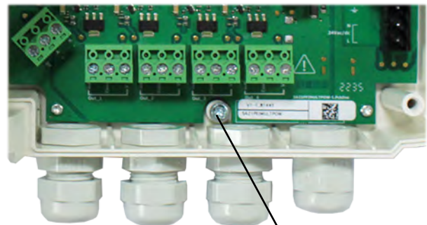
Vis de fixation du boîtier
